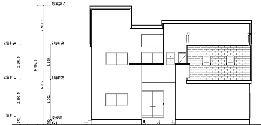
南側立面圖
