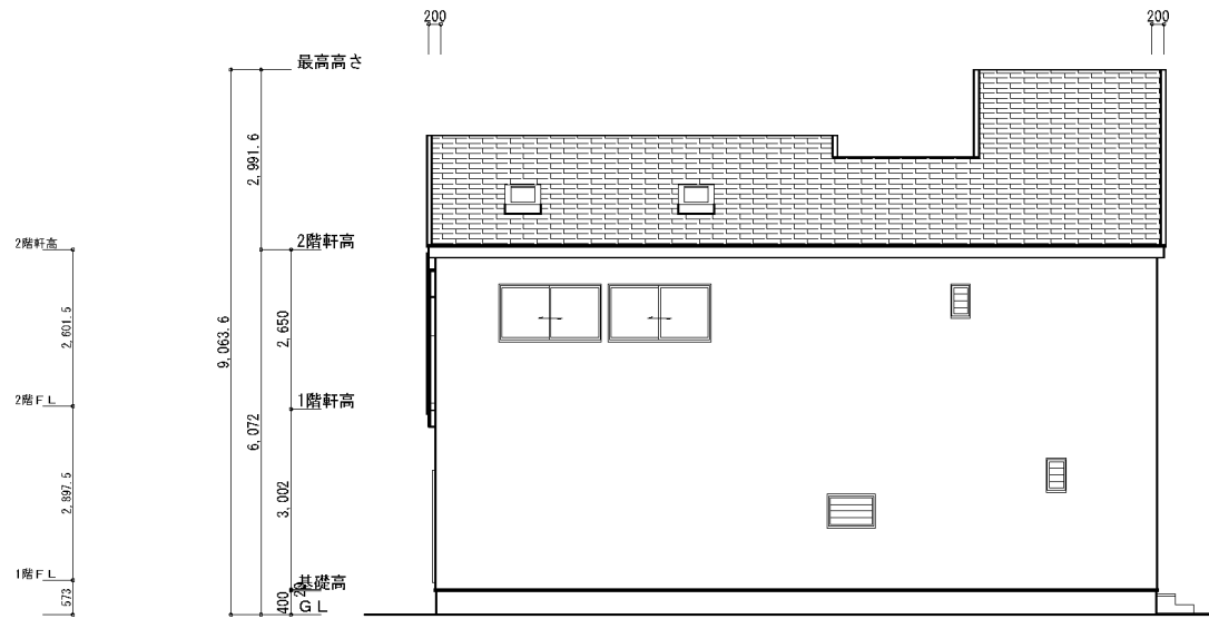
北側立面圖
