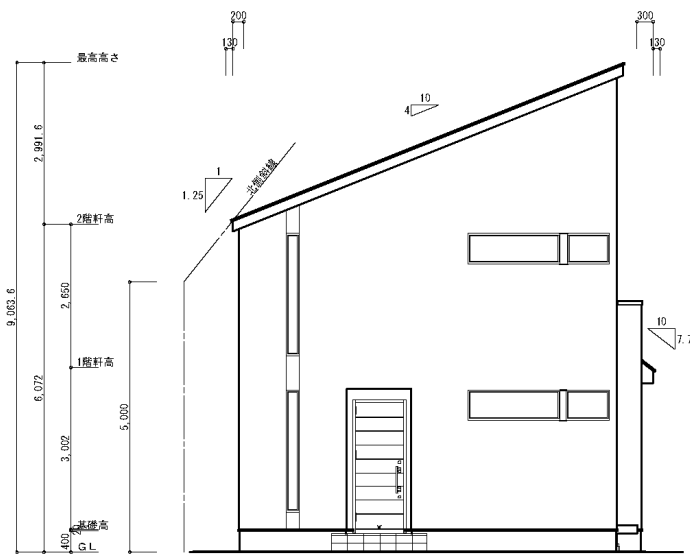
西側立面圖
