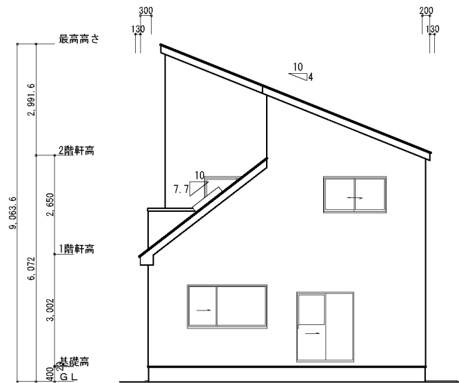
東側立面圖
