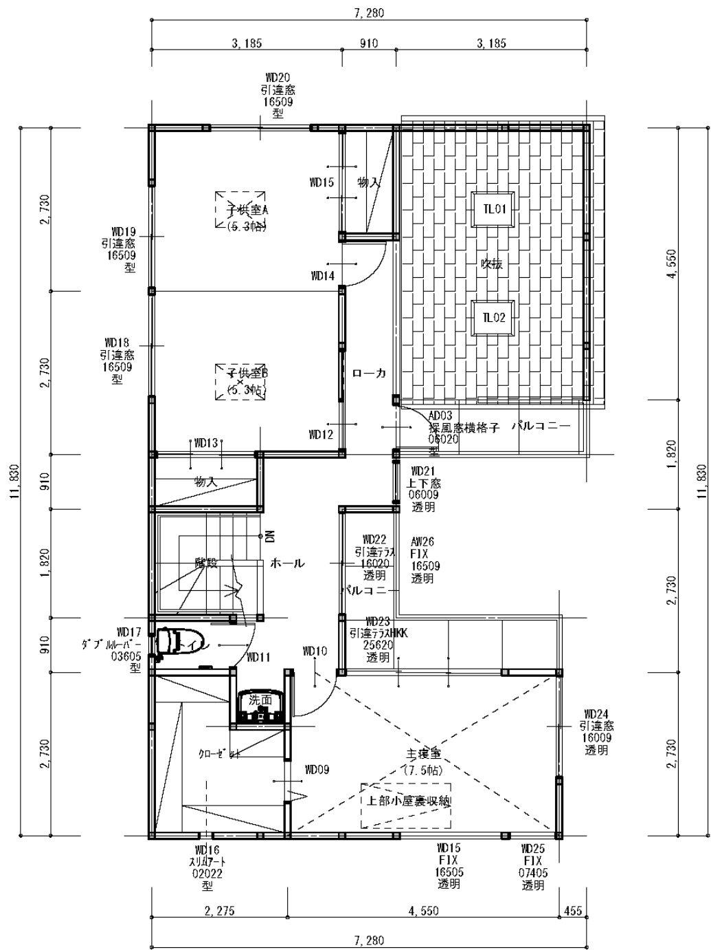
2階 平面図
