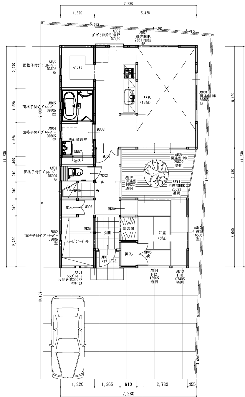
1階 平面図
