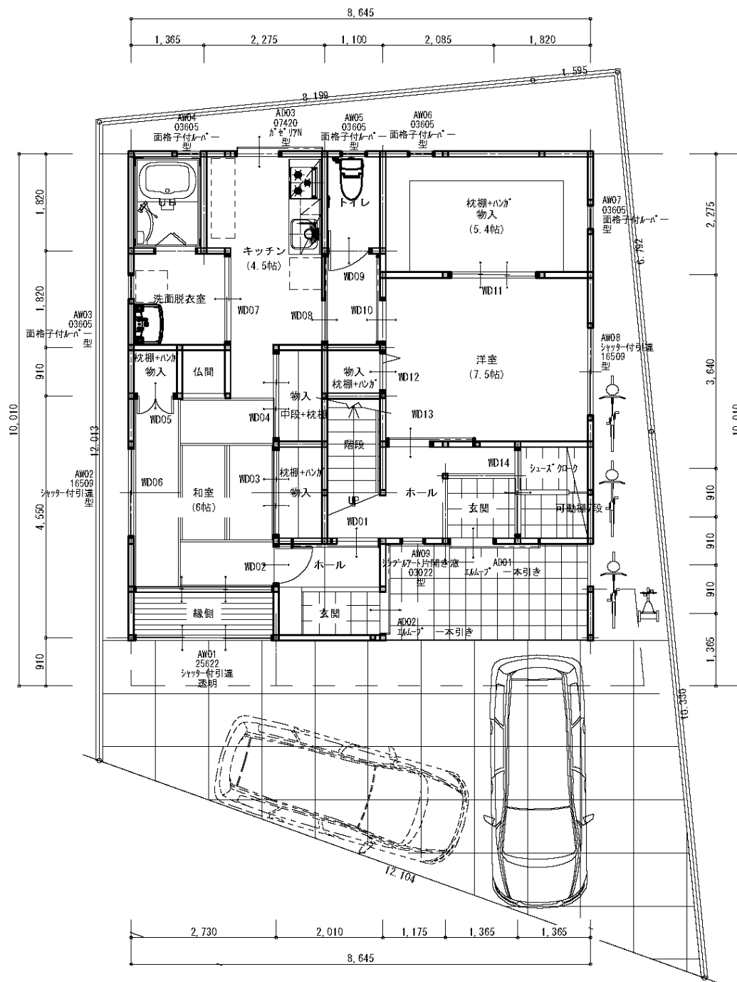
1階 平面図
