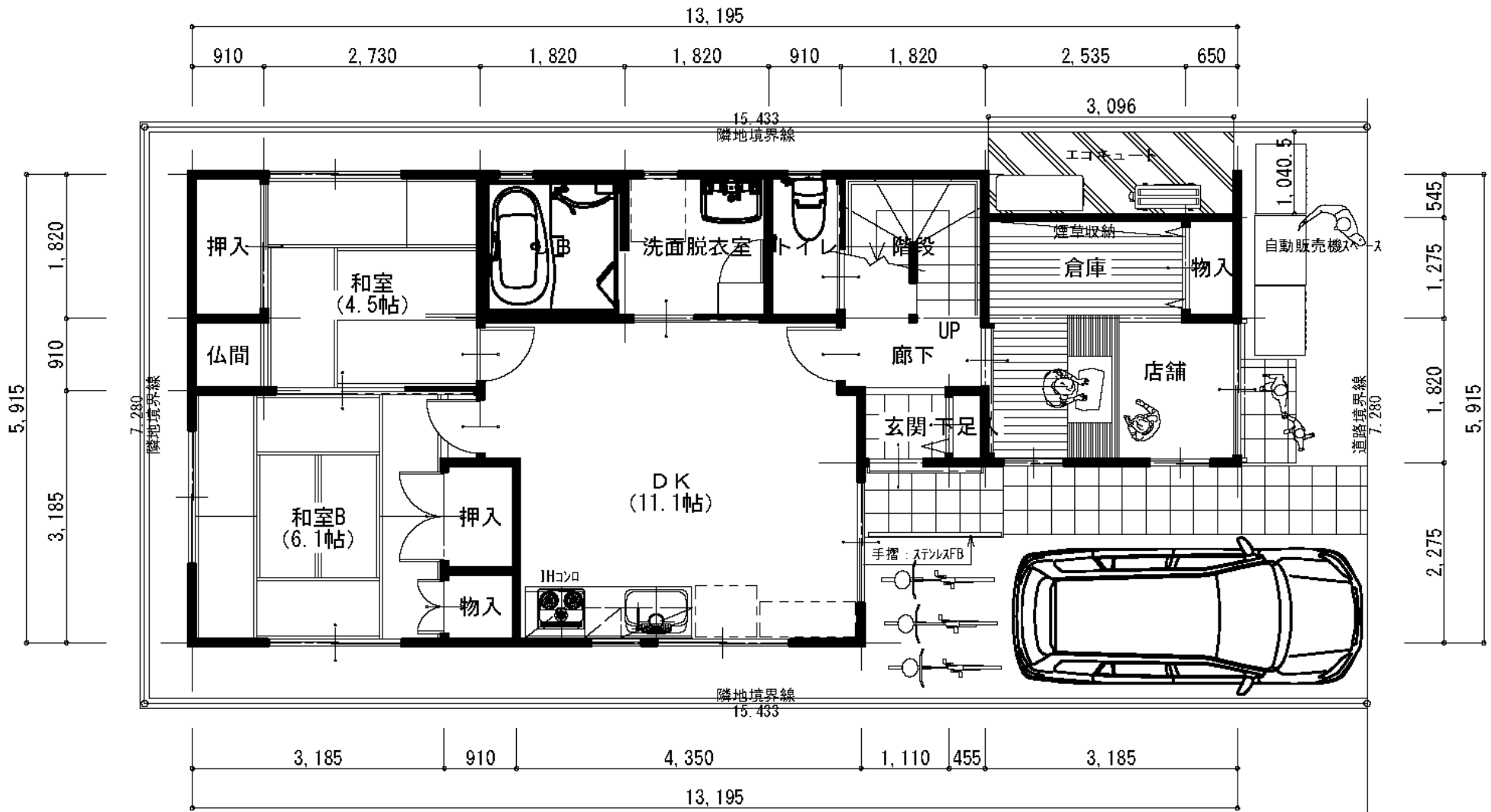
1階 平面図
