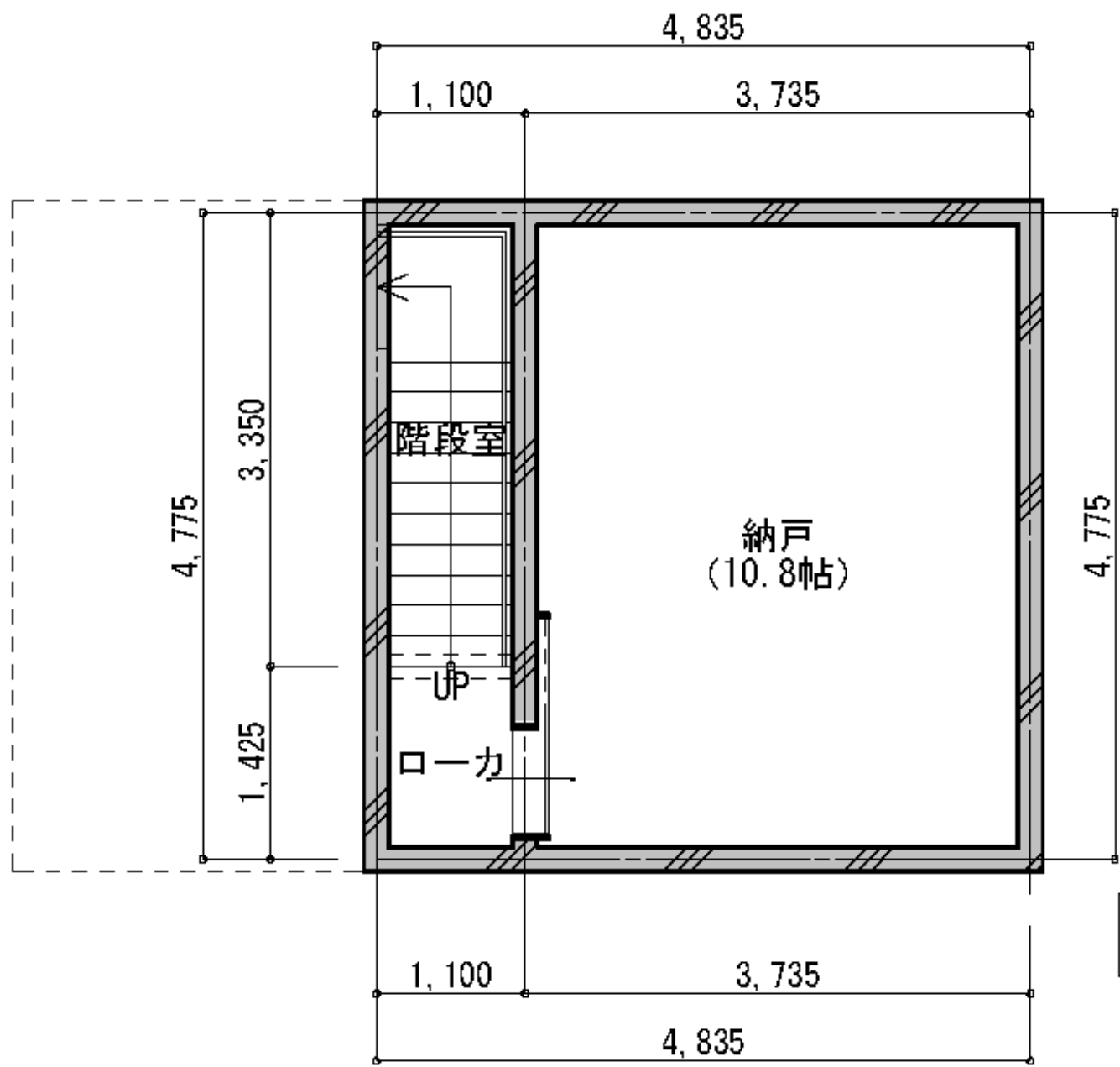
地下1階 平面図
